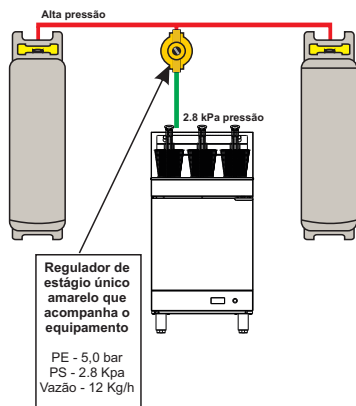
Instalação do Gás GLP - Com um equipamento na rede
