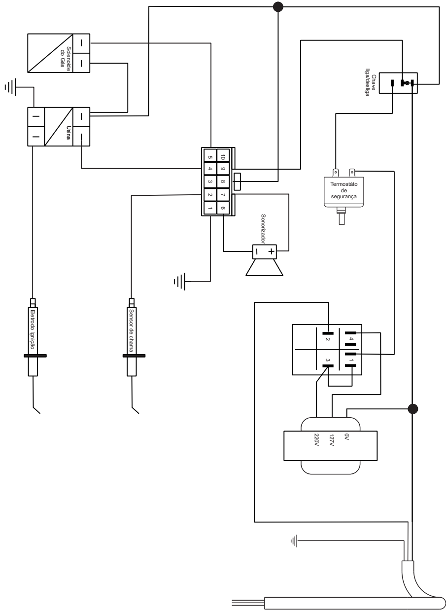
ESQUEMA ELÉTRICO FOG 2/3 C - Monofásico
